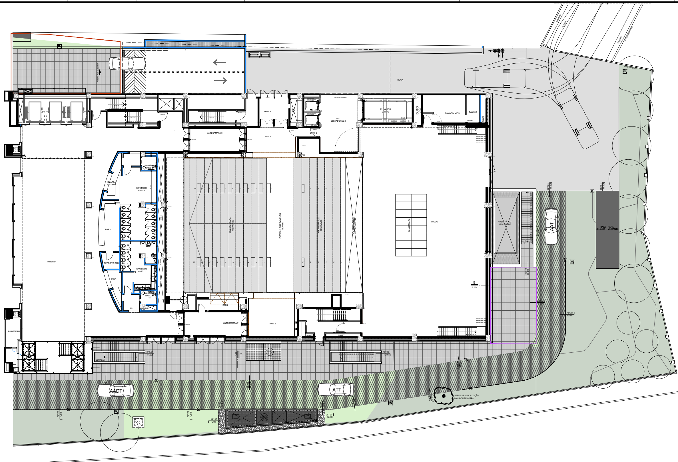
PLANTA DO PAVIMENTO TÉRREO ESCALA 1:100
